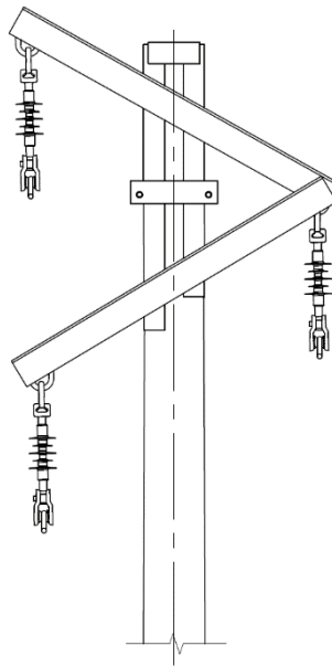
Рисунок 2.5.5.20 – Пример конструкции СВЛ
