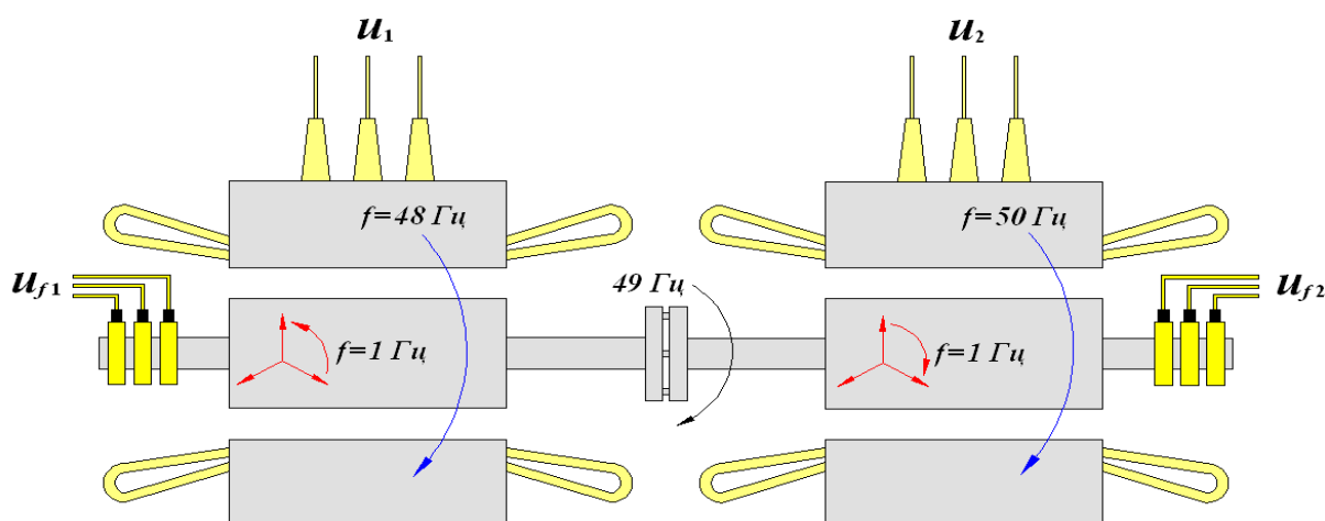
Рисунок 2.7.4.4 - Асинхронизированный электромеханический преобразователь (функциональная схема соединений)
