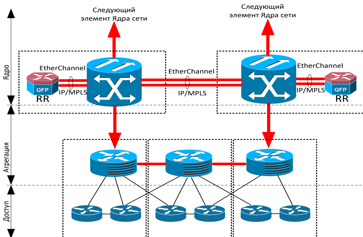
Рисунок 2.11.5.2 - Структура сети передачи данных ССЭСК
