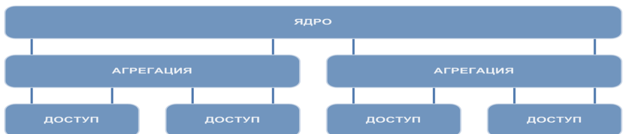
Рисунок 2.11.5.1 - Трехуровневая модель ССЭСК
