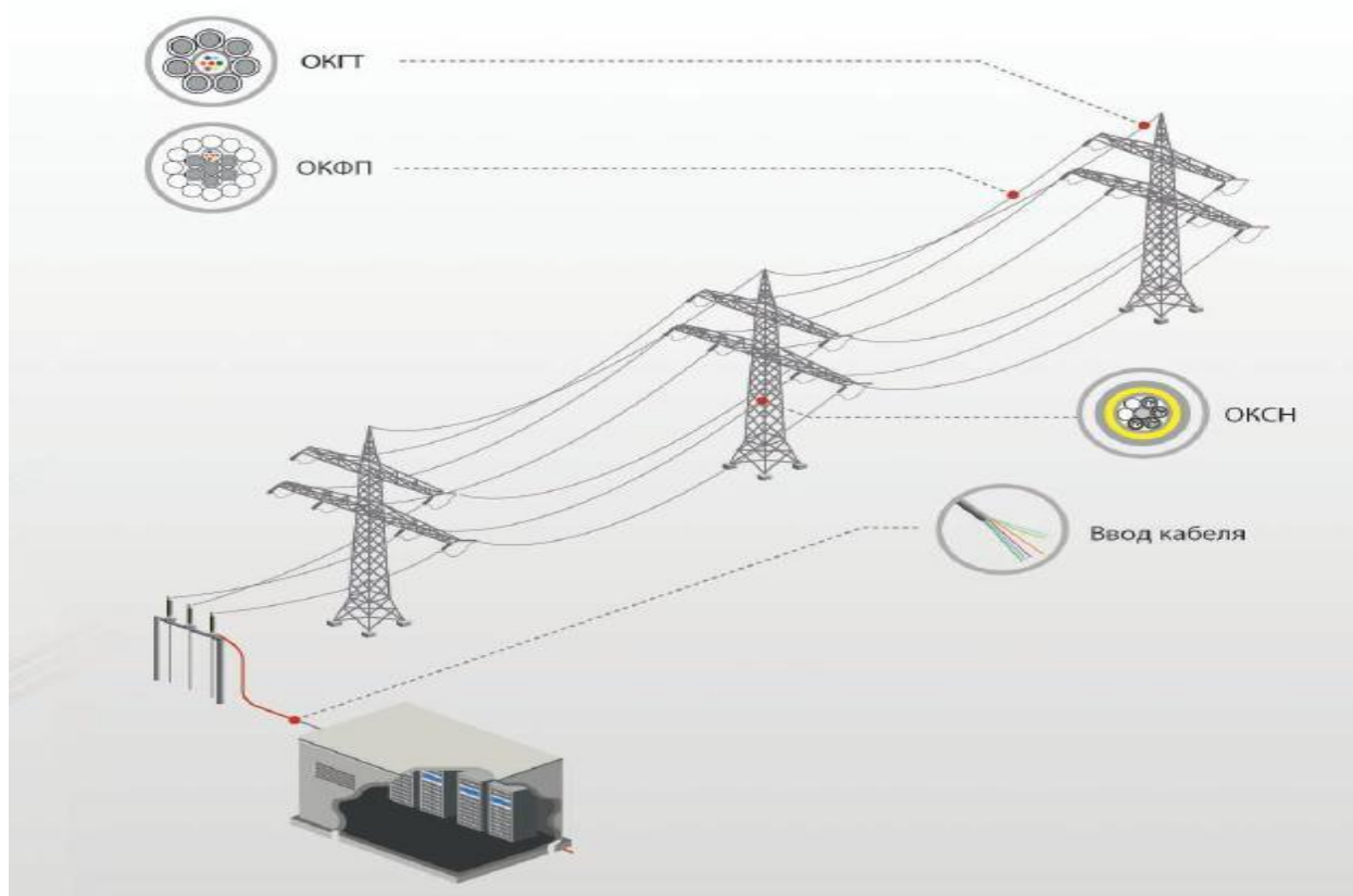
Рисунок 2.11.6.3.1 - Пример использования самонесущего кабеля (ОКСН) и оптического кабеля, встроенного в фазный провод (ОКФП) и грозозащитный трос (ОКГТ)
