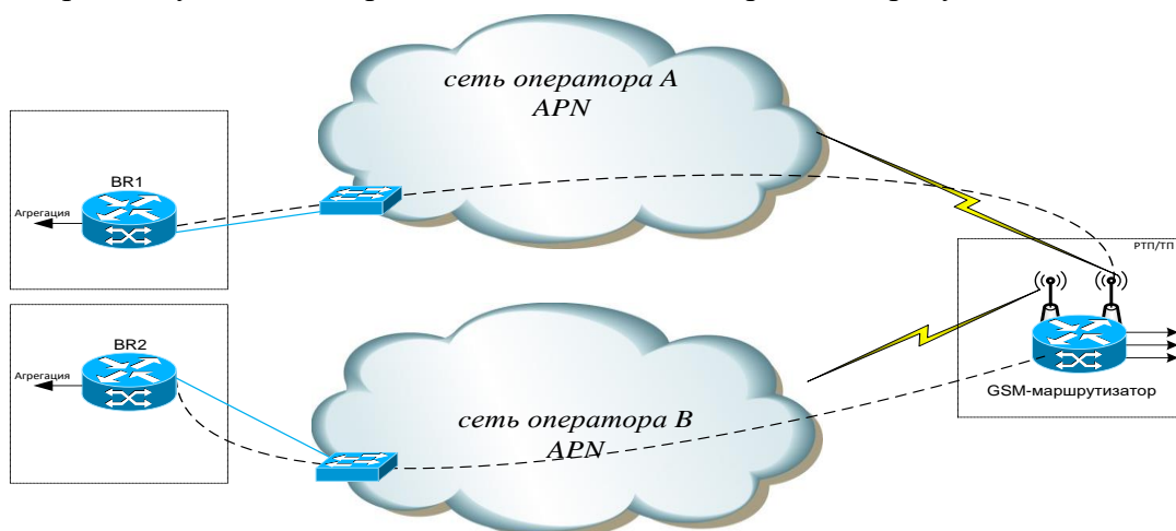
Рисунок 2.11.5.7.2 - Участок беспроводной сети по APN
