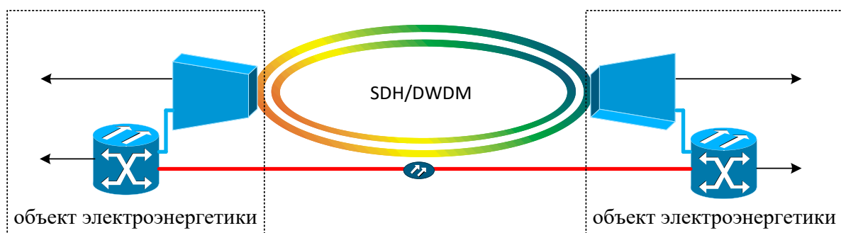
Рисунок 2.11.4.4 - Кольцевая архитектура ВОЛС
