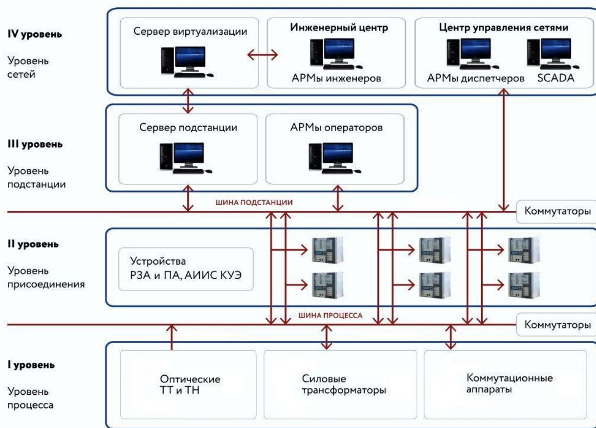
Рисунок 2.9.3.1 - Многоуровневая структура АСУ ТП
