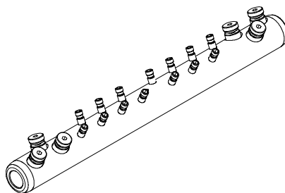
Рисунок 2.5.5.18 - Пример универсального зажима для ликвидации аварий на ВЛ 35-220 кВ
